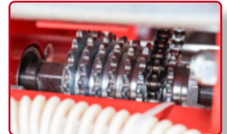
Sistema de transmisión de multivelocidad con 30 diferentes espacios entre fila y fila
