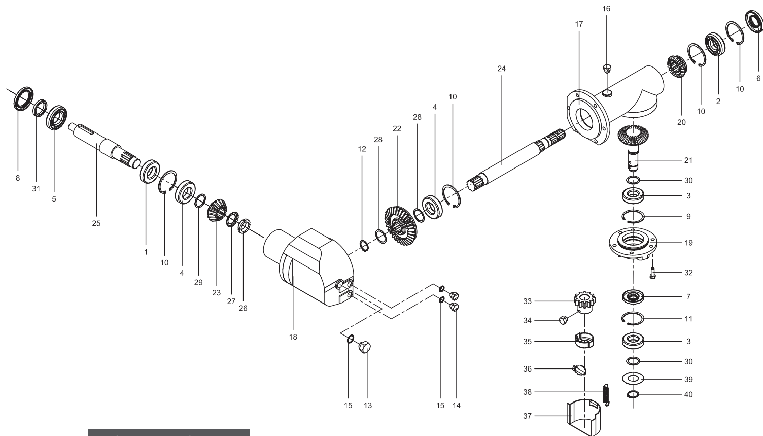
7.5 Gear Box / T-MSMHH-1.1.2
