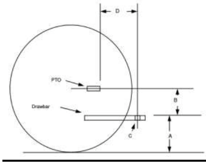
Figura 7- Las medidas y relaciones en los puntos B y D para el Mezclador-Alimentador Vertical Minos . La toma de fuerza del tractor y la posición de la barra de tiro están diseñadas con medidas específicas para el tamaño y la potencia nominal del tractor. (Figura 8) El operador no debe realizar cambios en estos estándares de diseño cambiando el punto de enganche. La Tabla 8 enumera las medidas y relaciones en los puntos A, B, C y D para cada rango de tamaño de tractor.
