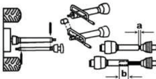
Figura 12- Ajuste del eje de la toma de fuerza a la longitud adecuada
