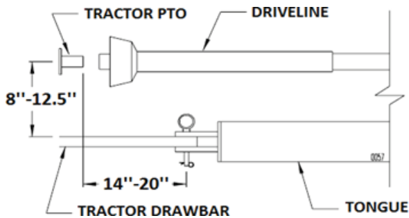
Figura 7- Las medidas y relaciones en los puntos B y D para el Mezclador-Alimentador Vertical Minos . La toma de fuerza del tractor y la posición de la barra de tiro están diseñadas con medidas específicas para el tamaño y la potencia nominal del tractor. (Figura 8) El operador no debe realizar cambios en estos estándares de diseño cambiando el punto de enganche. La Tabla 8 enumera las medidas y relaciones en los puntos A, B, C y D para cada rango de tamaño de tractor.
