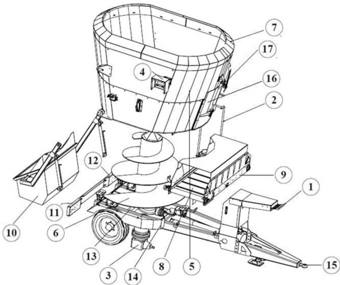
Figura 2- Partes principales de la máquina
