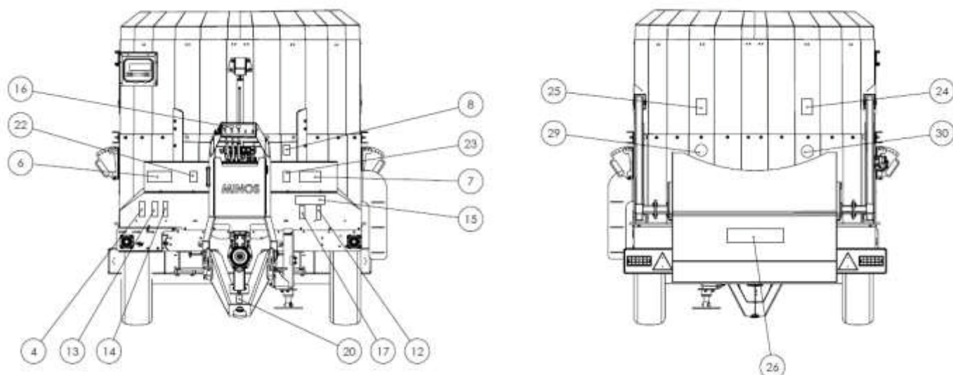
Figura 3.1 Posición en la máquina de las calcomanías de seguridad con textos de advertencia (dibujo)
