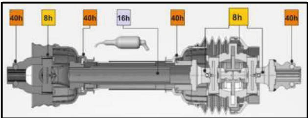
Figura 27- Los Puntos de lubricación.
