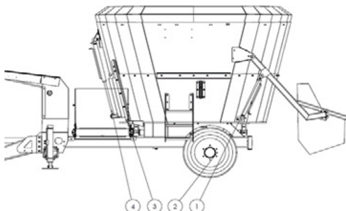
Figura 22- Los puntos de lubricación en el mezclador.
