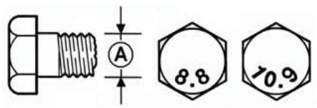
Figura 21- tamaño de la rosca(A)
