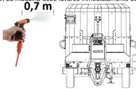
Figura 28- Distancia segura entre el chorro de agua y el mezclador-alimentador.
