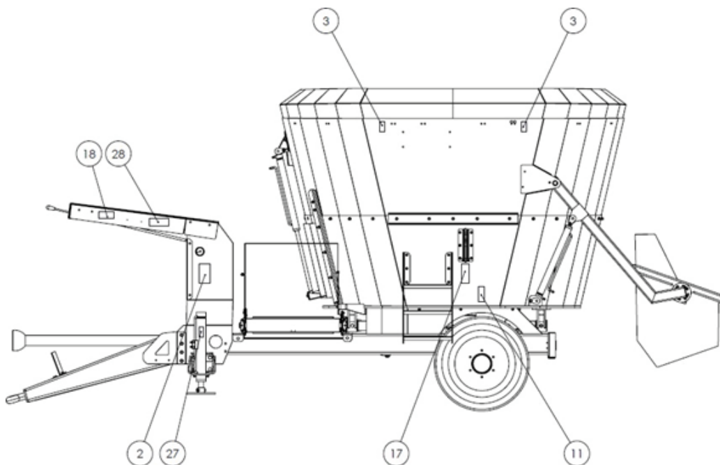
Figura 3.2- Posición en la máquina de las calcomanías de seguridad con texto de advertencia
