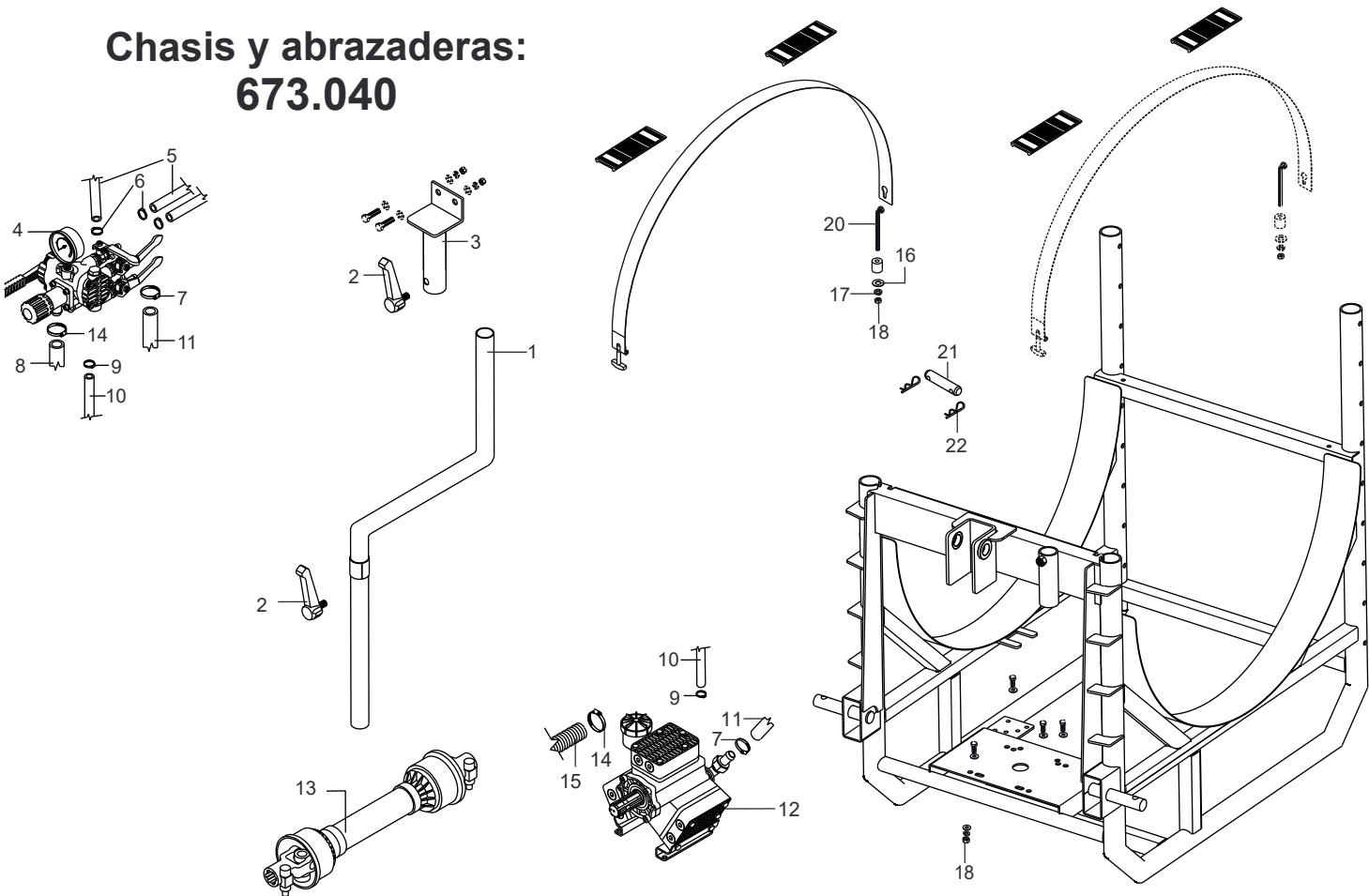
Chasis y abrazaderas equipo 673.040
