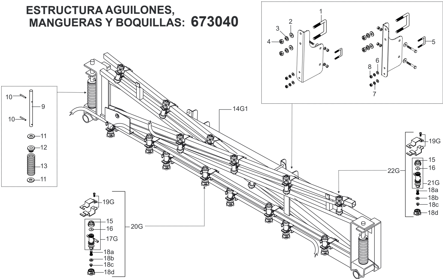
ESTRUCTURA DE AGUILONES, MANGUERAS Y BOQUILLAS 673040
